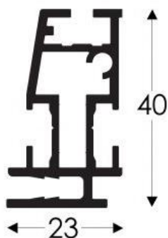
obr. 01 – řez hliníkovým profilem
