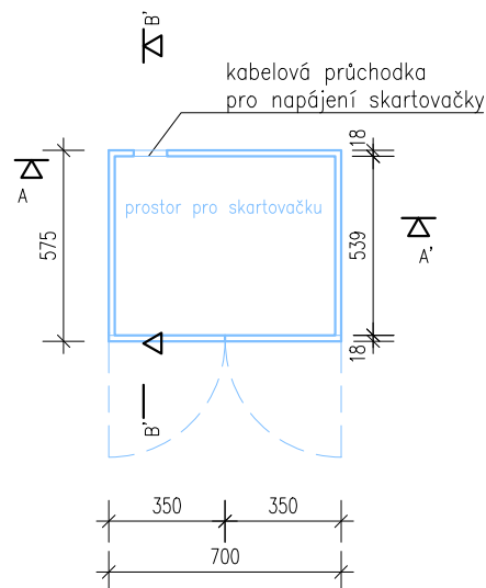
PŮDORYSNÝ ŘEZ VE VÝŠCE 150 mm
