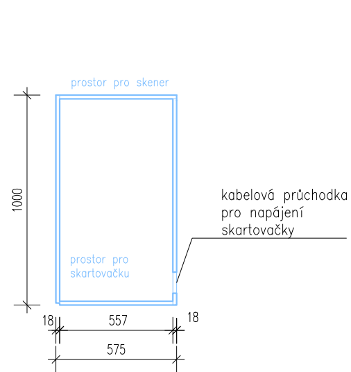
ŘEZ B-B'
