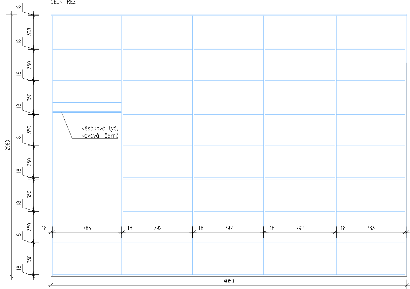
ČELNÍ ŘEZ
