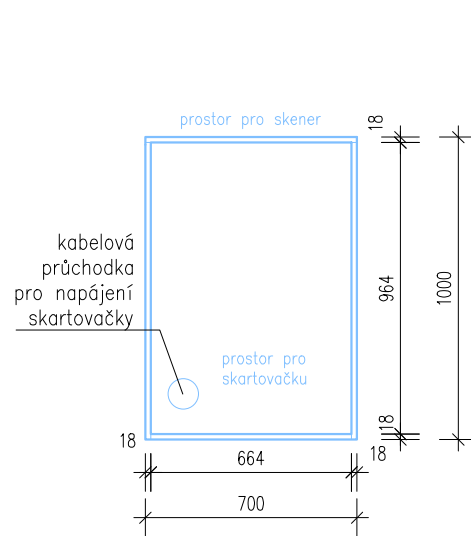
ŘEZ A-A'
