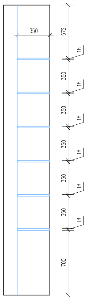
BOČNÍ ŘEZ
