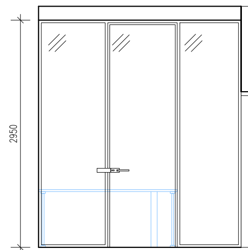
POHLED NA STĚNU A
