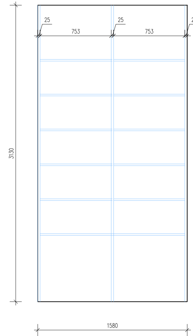
ČELNÍ POHLED
