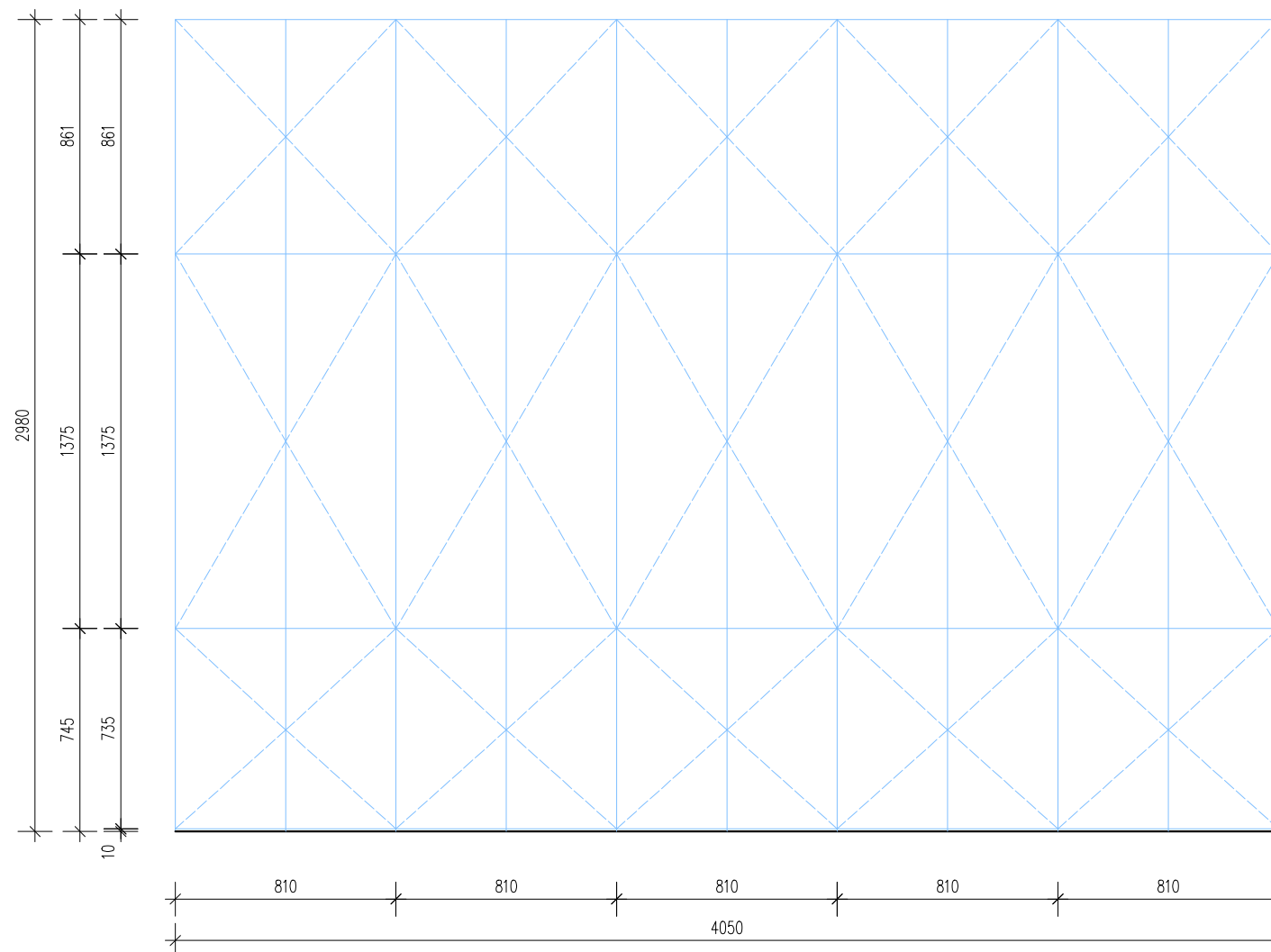
ČELNÍ ŘEZ
