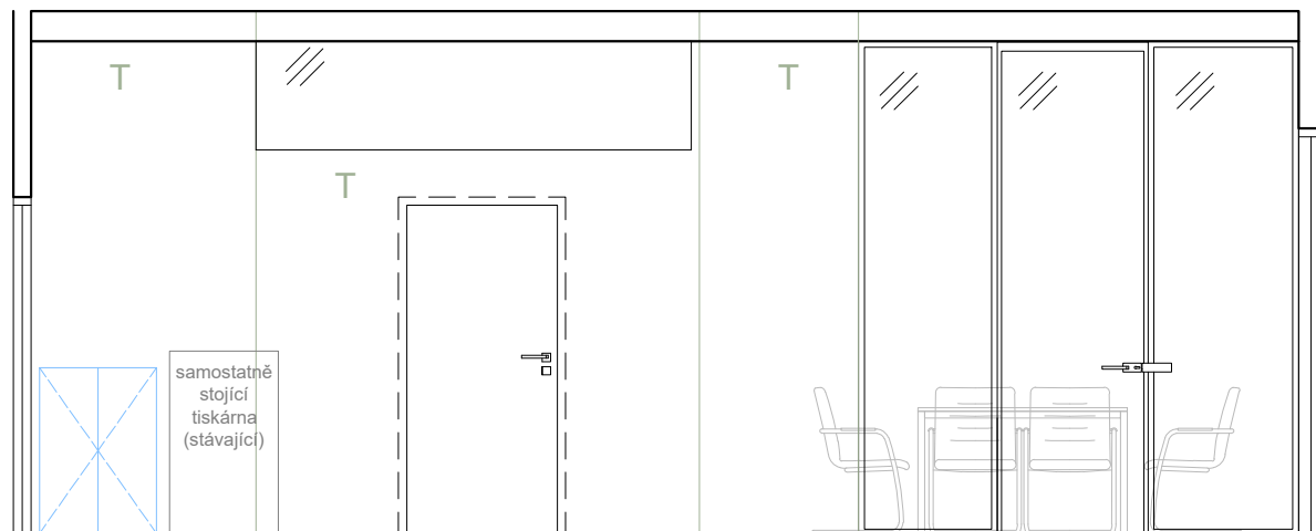
POHLED NA STĚNU C
