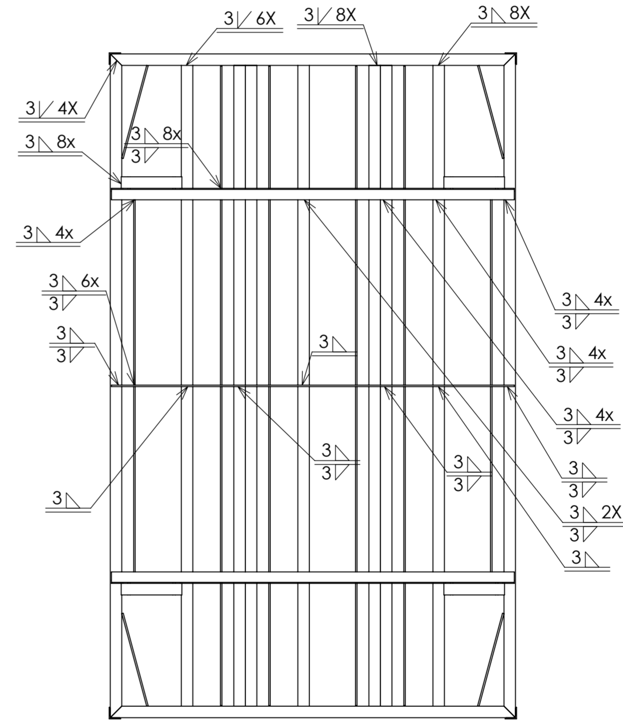
POHLED D MĚŘITKO 1 : 10
